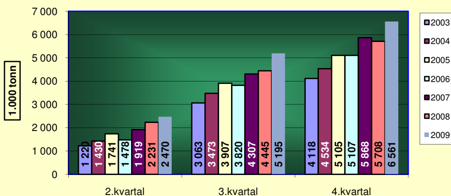
Produksjon av varme og halvvarme asfaltmasser i Norge
